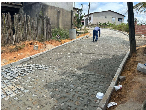
FOTO 11: PAVIMENTAÇÃO EM PARALELEPÍPEDOS GRANÍTICOS EXECUTADA;
